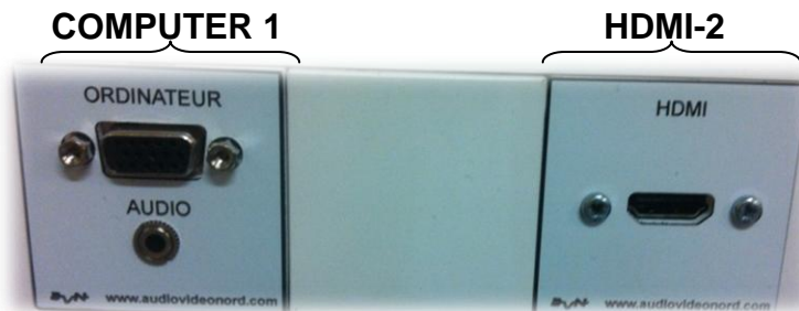
Figure 4: Prises VGA (à gauche) et HDMI (à droite) fixées au mur
